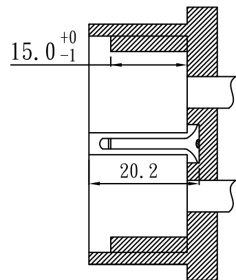
A--A(Broken)
