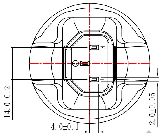
A--A(Broken)
